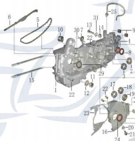
Motorgehäuse links mit Getriebeglocke
