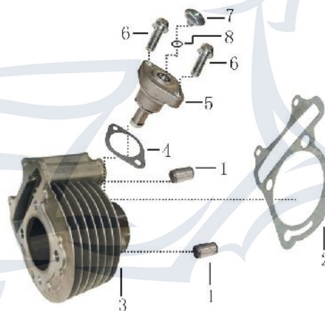
Zylinder / Kettenspanner
