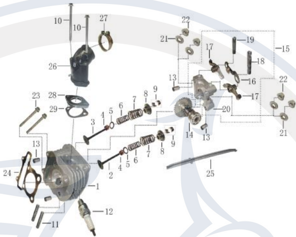
Zylinderkopf ohne SLS / Nockenwelle und Ansaugstutzen - GY6-2
