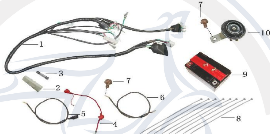
Kabelbaum / Schlossatz / Batterie
