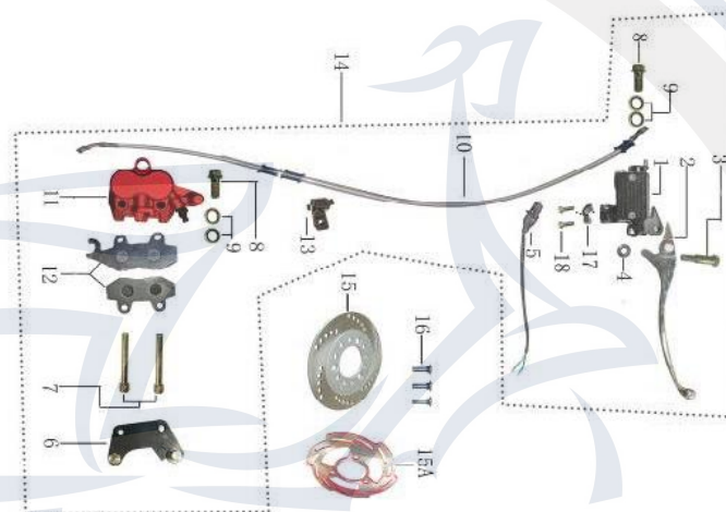
Bremsanlage vorne
