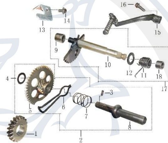
Kickstarter und Freilauf
