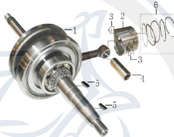
Kurbelwelle mit Kolben
