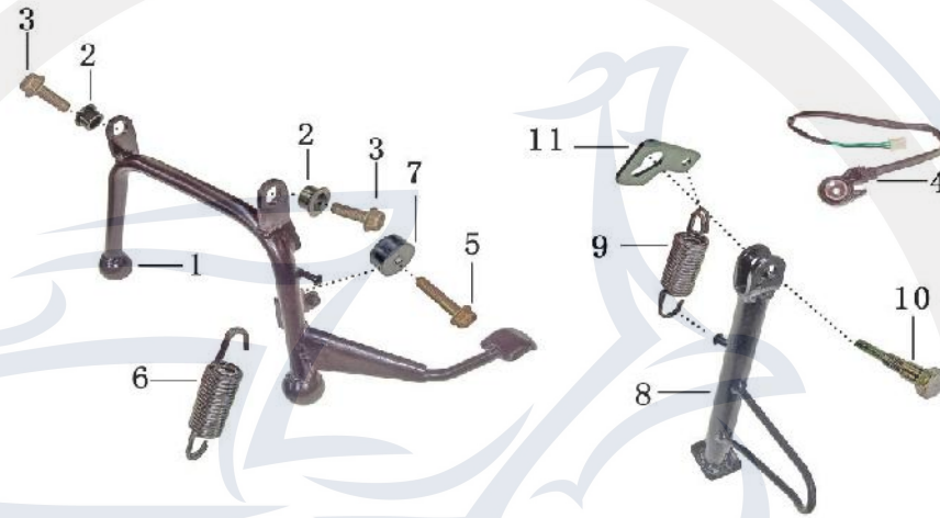
Hauptständer und Seitenständer mit Schalter
