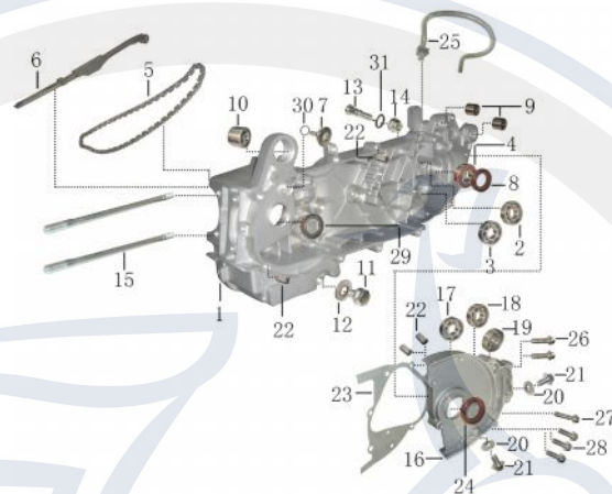
Motorgehäuse links mit Getriebeglocke
