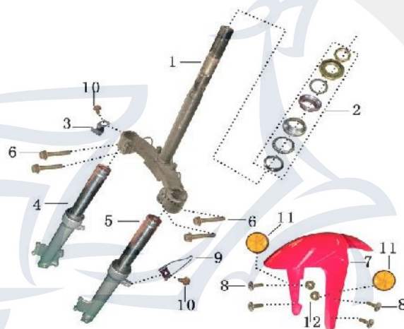
Vorderradgabel mit Schutzblech
