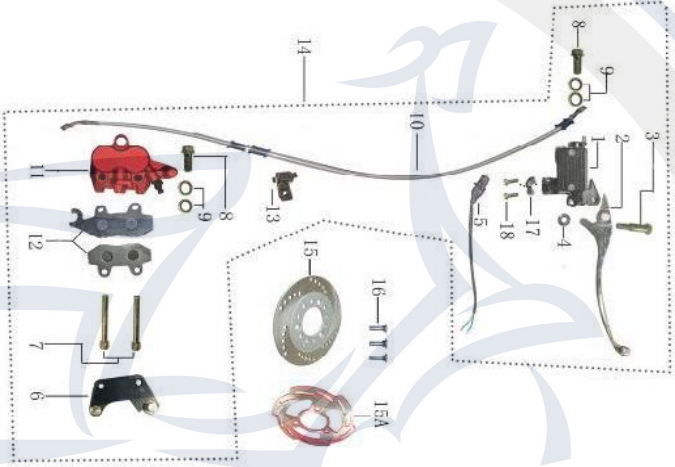
Bremsanlage vorne
