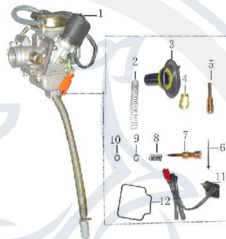
Vergaser ( HL IC PD24J)
