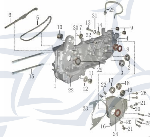
Motorgehäuse links mit Getriebeglocke
