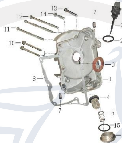
Gehäusedeckel rechts mit Ölsieb
