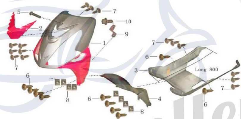
Frontverkleidung - Firejet 125 Unterfahrschutz
