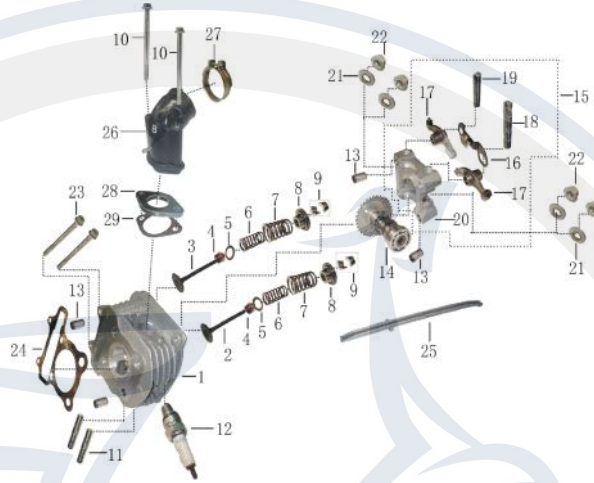
Zylinderkopf ohne SLS / Nockenwelle und Ansaugstutzen - GY6-2
