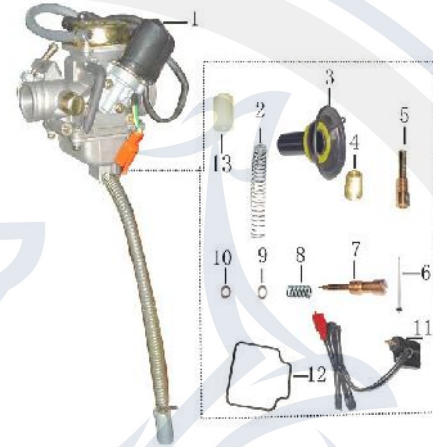
Vergaser (KF CV PD24J)
