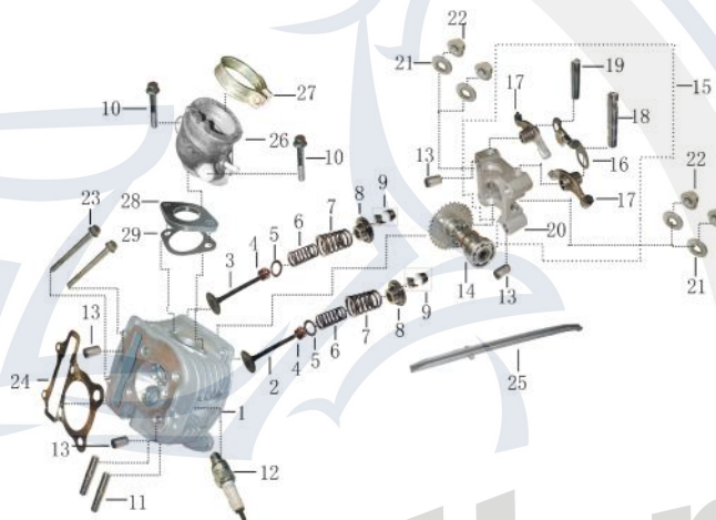
Zylinderkopf ohne SLS / Nockenwelle und Ansaugstutzen - GY6-1
