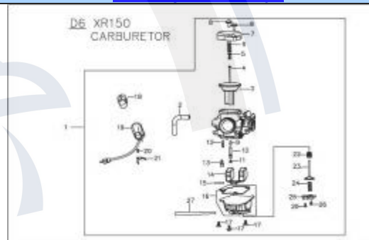
D6 - Vergaser
