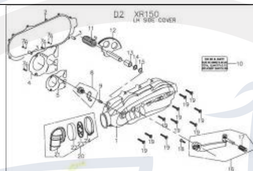
D2 - Linke Seitenabdeckung
