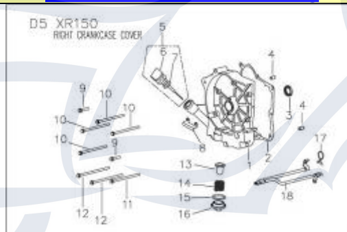
D5 - Rechte Kurbelgehäuseabdeckung
