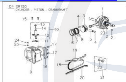
D4 - Kurbelwelle
