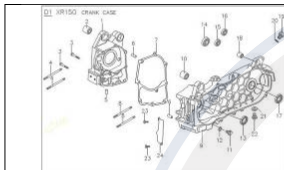
D1 - Rechtes Kurbelgehäuse
