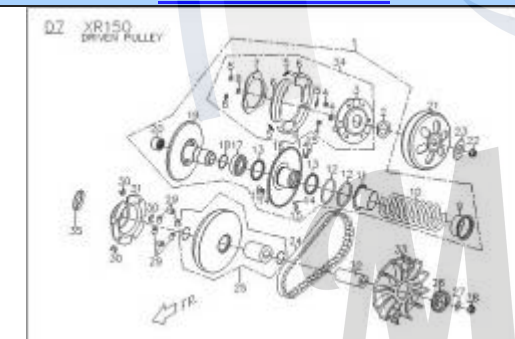
D7 - Riemenscheibe
