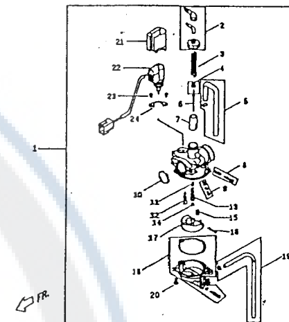
E9 化油器 CARBURETOR
