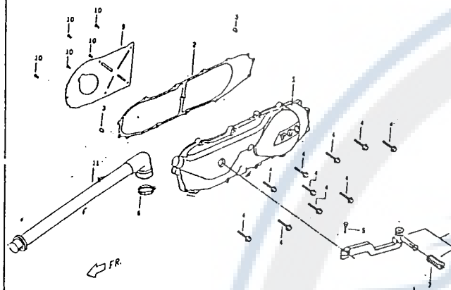
E7 左邊蓋 LH SIDE COVER
