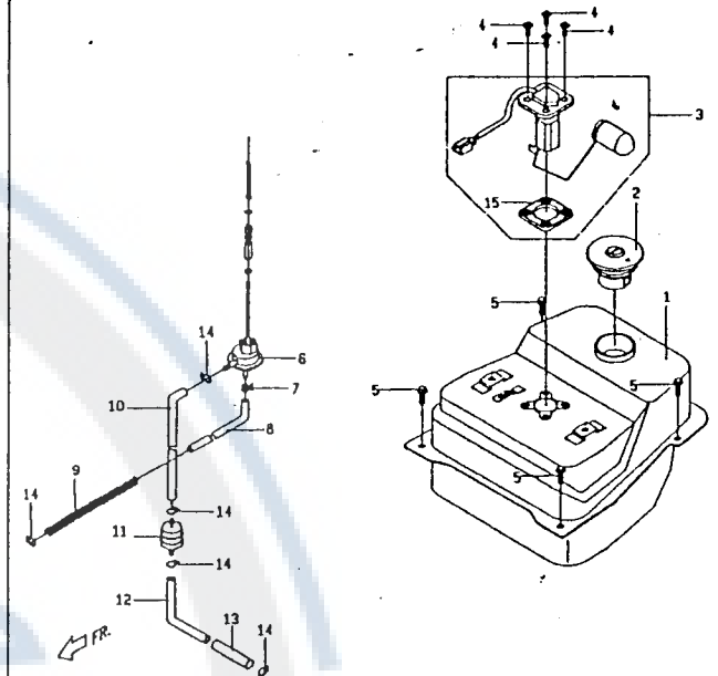
F15 汽油箱 FUEL TANK
