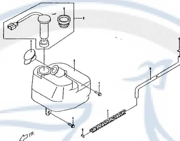
F14 機油箱 OIL TANK
