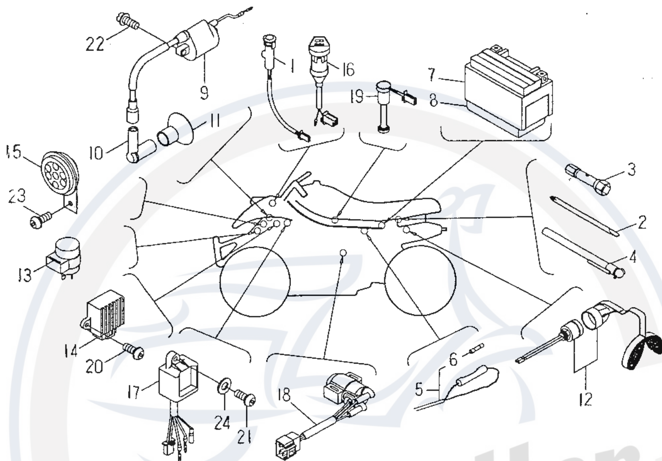
FIG.29 WIRE HARNESS 主電路配線
