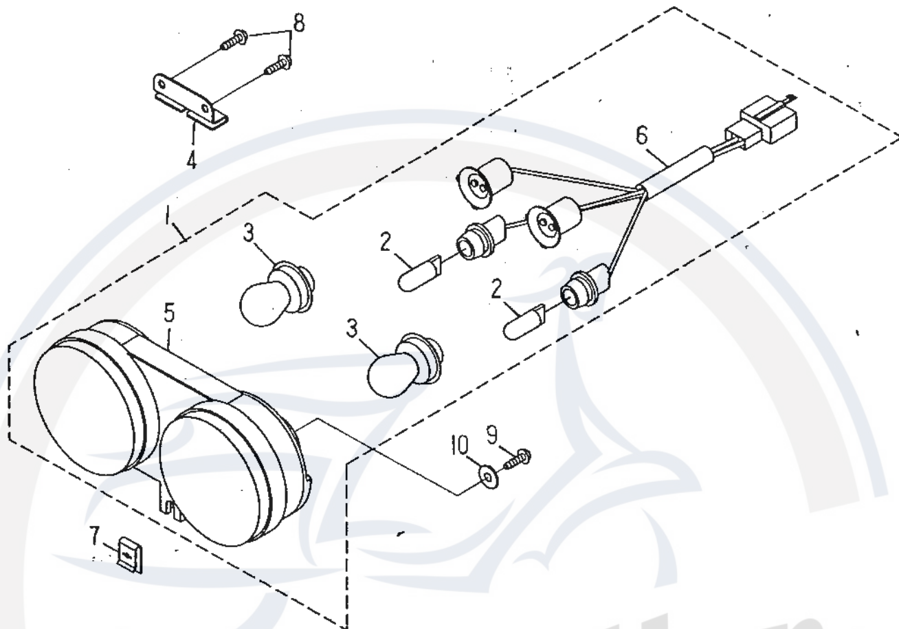
FIG.31 HEAD LIGHT 前燈
