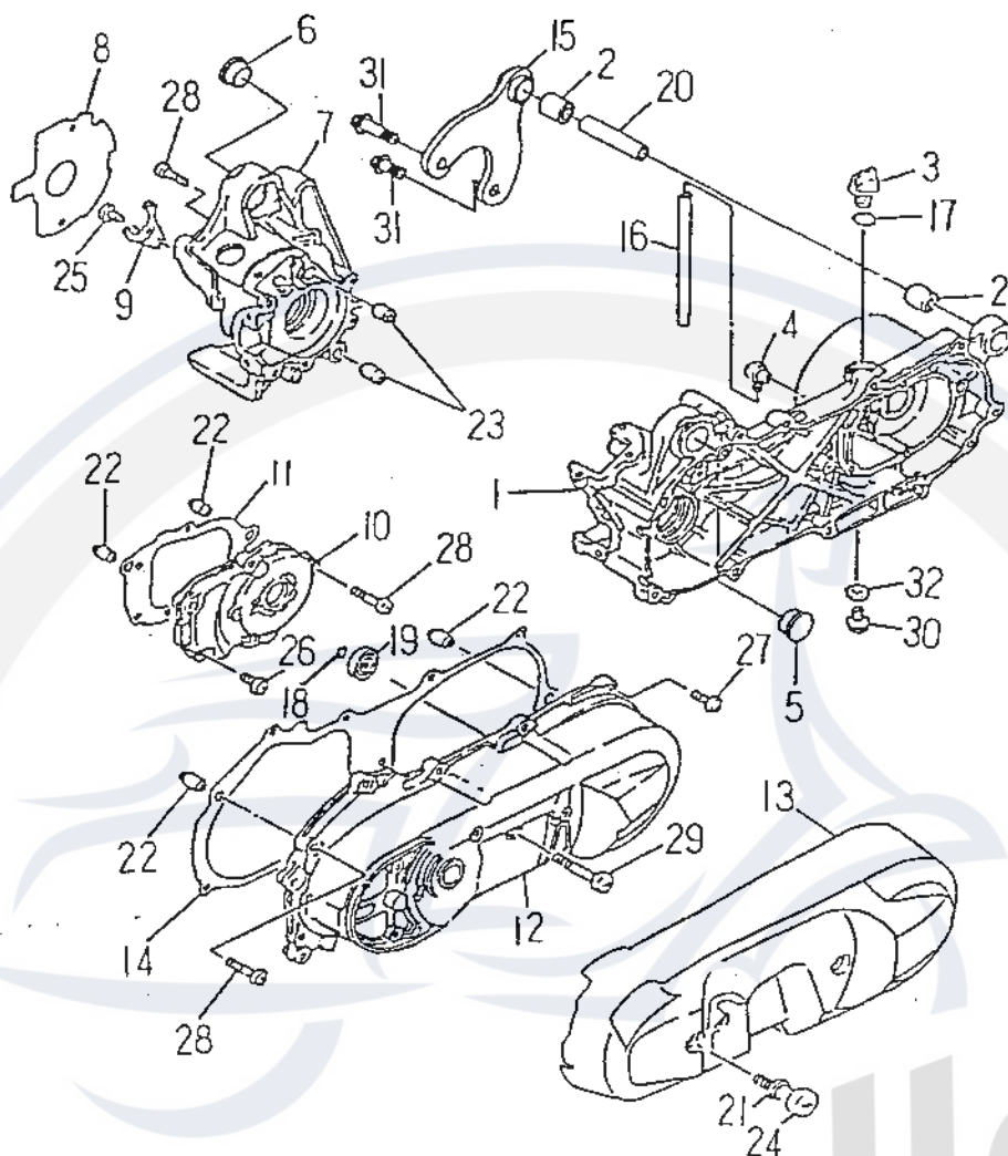
FIG.07 CRANKCASE 曲軸箱
