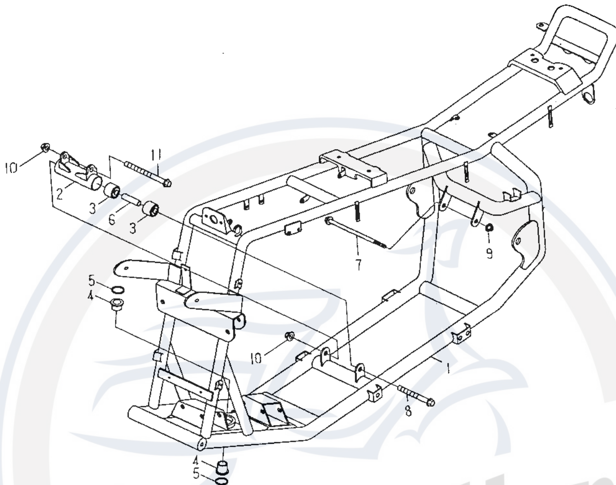
FIG.16 FRAME 車架
