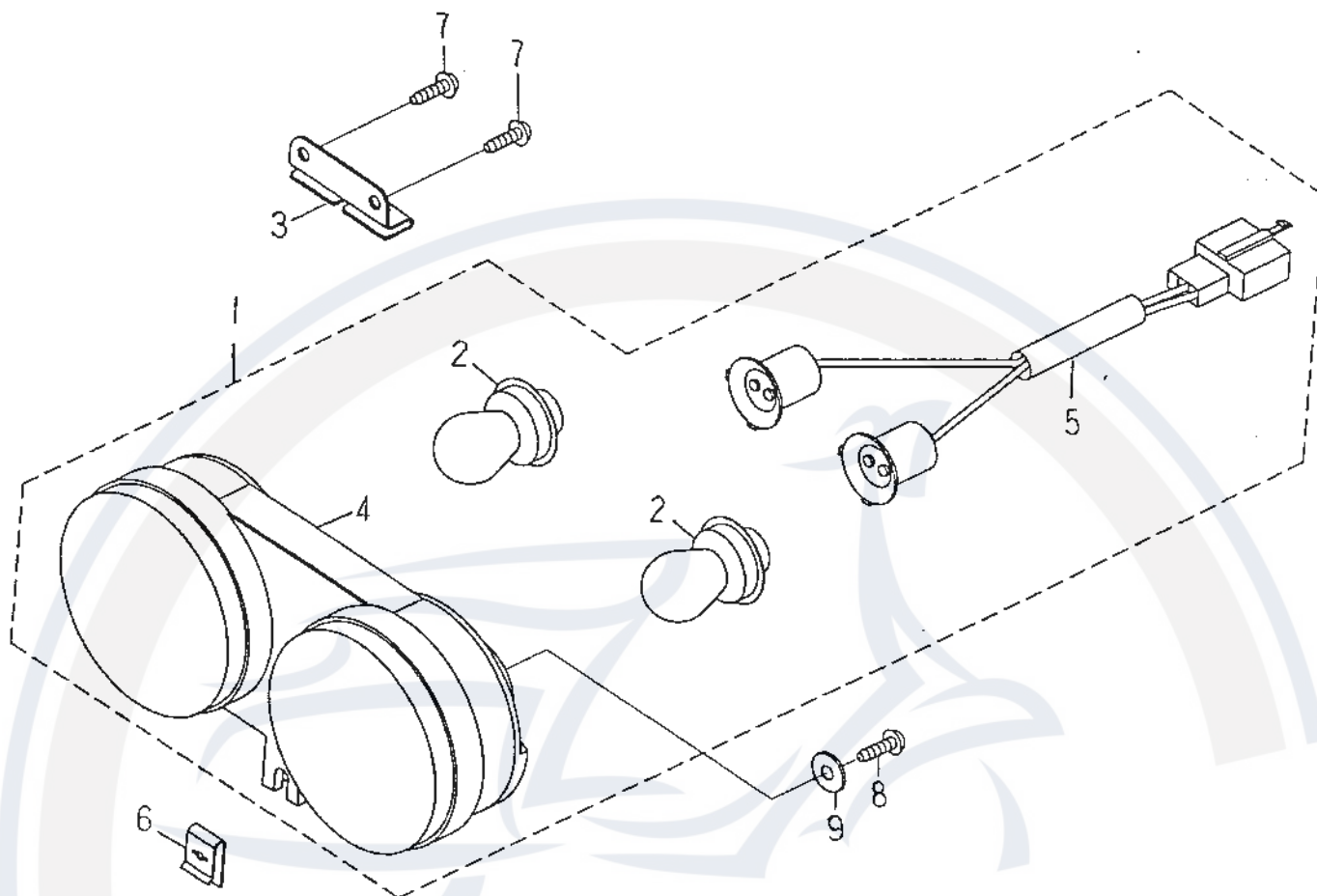
FIG.31 HEAD LIGHT 前燈
