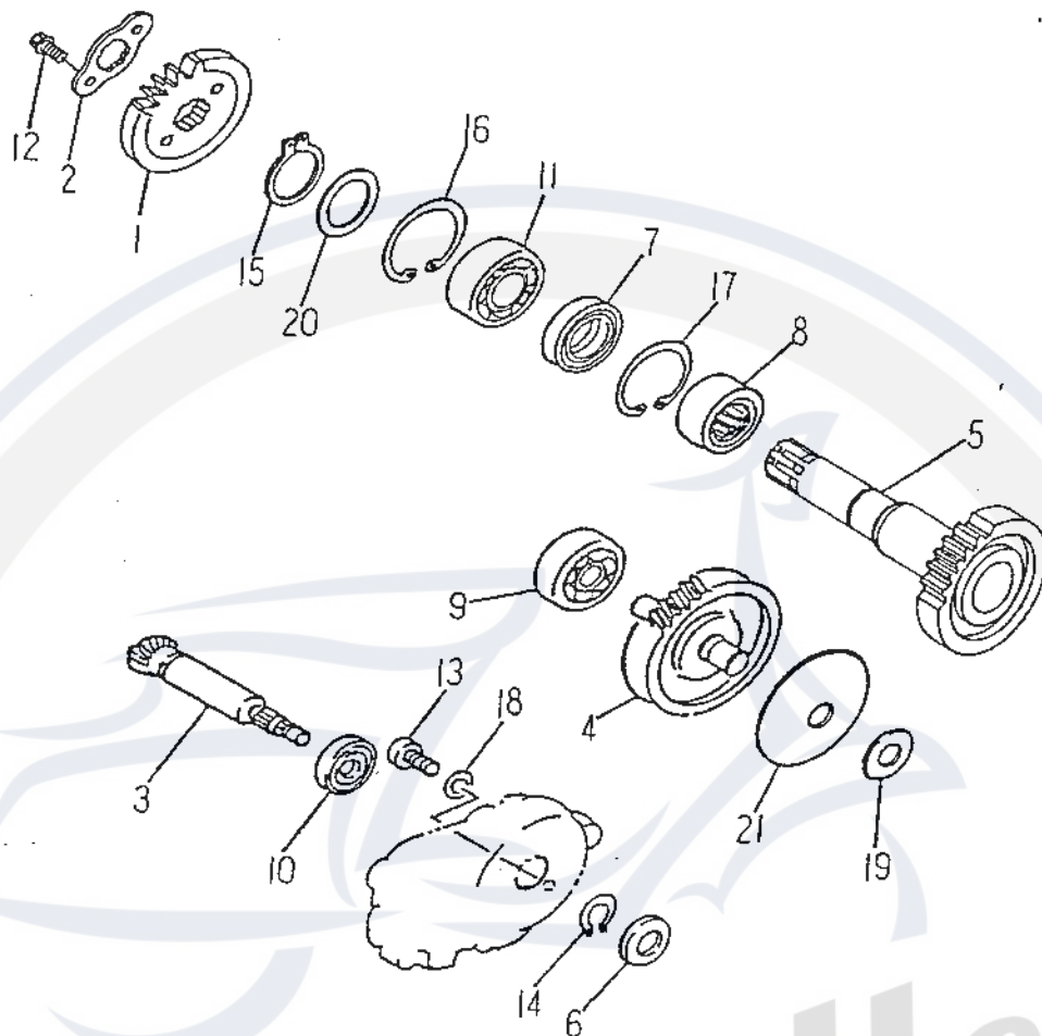
FIG.10 TRANSHISSION 傳動機構
