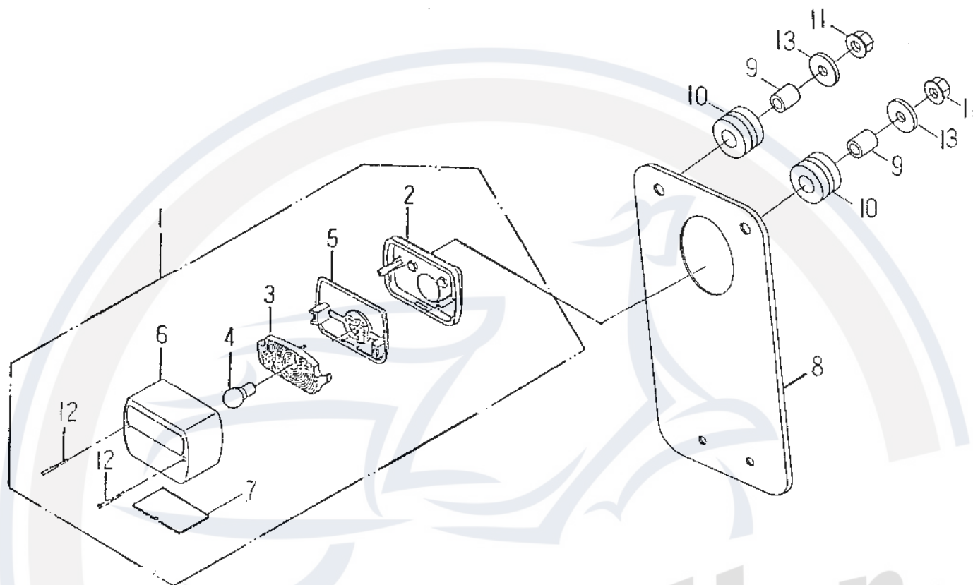
FIG.32 TAIL LIGHT 後燈
