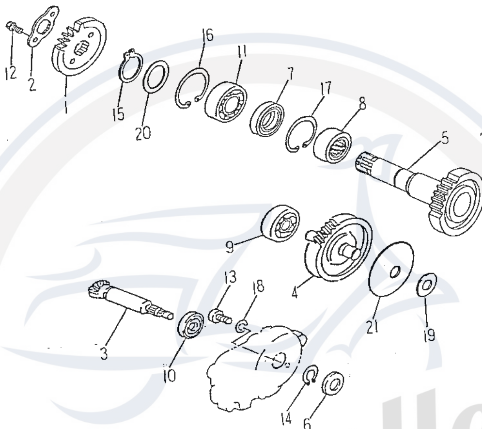
FIG.10 TRANSMISSION 傳動機構
